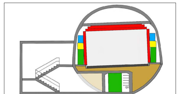
Skizze der Varianten 2 und 3: Fluchtweg durch Sicherheitsstollen. Varianten sind spiegelbildlich zueinander. Eigene Darstellung
