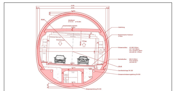
Normalprofil des Tunnels, bestimmt im Rahmen dieser Bachelorarbeit. Eigene Darstellung
