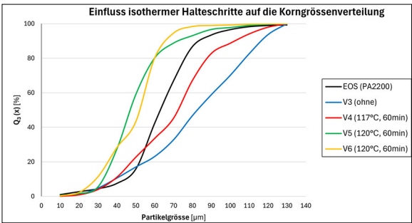
Abb. 1: Analyse des hergestellten Pulvers anhand der Korngrössenverteilung Eigene Darstellung
