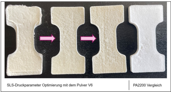
Abb. 3: Zugstäbe aus dem SLS-Forschungsdrucker, aus dem hergestellten PA12-Pulver Eigene Darstellung
