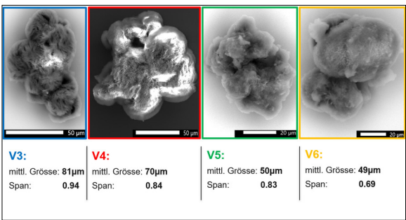
Abb. 2: Analyse der Kornform und Oberflächenstruktur mittels REM-Aufnahmen Eigene Darstellung
