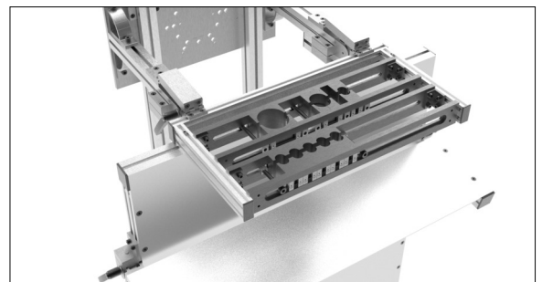
Modularer Klemmblock zur Fixierung von Kabeln Eigene Darstellung
