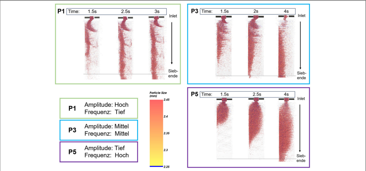
Graphische Auswertung der Produktverteilung auf dem Sieb und der Produktgeschwindigkeit über dem Sieb. Eigene Darstellung
