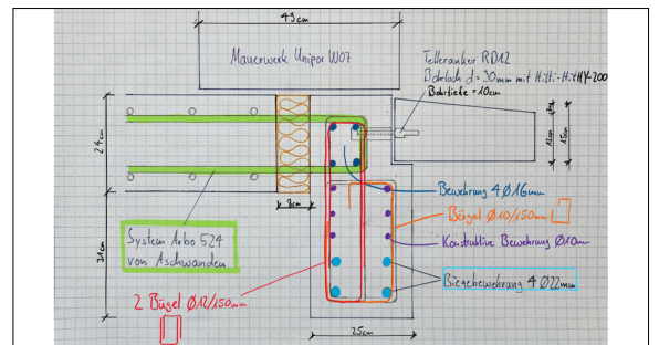
Abb. 2: Anschlussdetail Unterzüge an Ortbetondecke mit thermischer Trennung und Abfangung der Mauerwerkswand Eigene Darstellung
