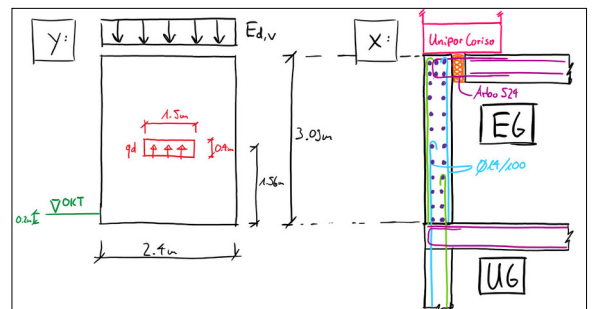
Abb. 3: System der massgebenden Wandscheibe für Anprall mit separater Federsteifigkeitsberechnung Eigene Darstellung
