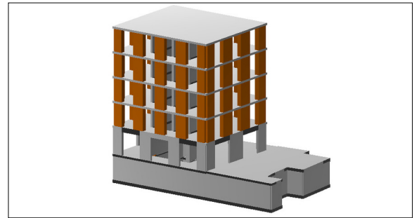
Abb. 1: Gerendertes Plattenstapelmodell aus Cedrus-8 Eigene Darstellung
