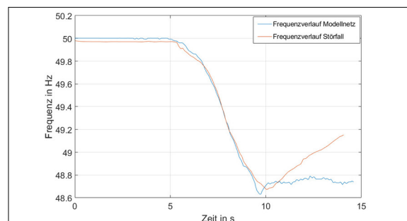
Gegenüberstellung Frequenzverlauf Modellnetz und Störfall Eigene Darstellung
