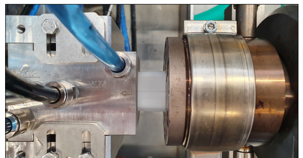
Abb.3: Einzug des extrudierten Profils in die Kalibrierung Eigene Darstellung
