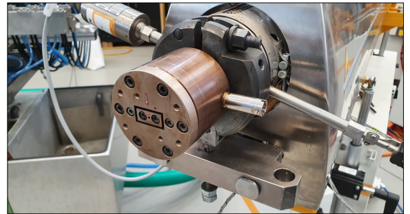
Abb.1: Extrusionswerkzeug Eigene Darstellung
