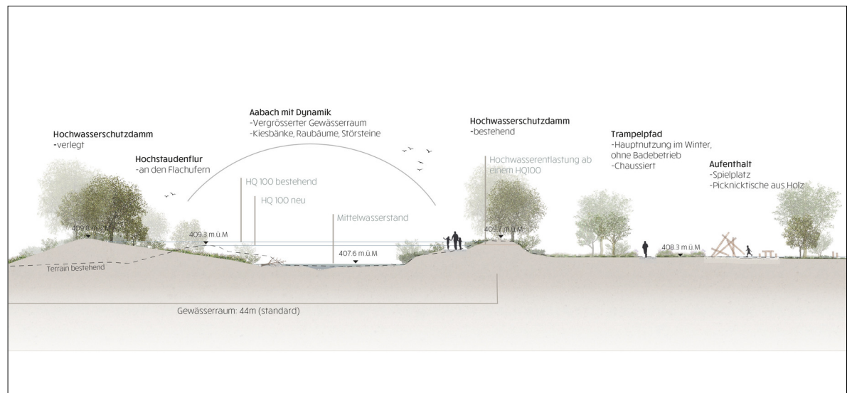
Schnitt durch die Parklandschaft mit Dammverlegung und Gewässerraumverbreiterung Eigene Darstellung
