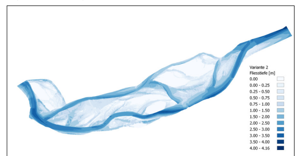
Resultat 2D - Simulation Variante 2 mit HQ5 - Fliesstiefen Eigene Darstellung
