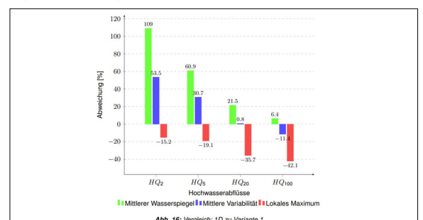
Vergleich der Wasserspiegellagen der 1D-Berechnung zur Variante 1 der 2D-Berechnung Eigene Darstellung
