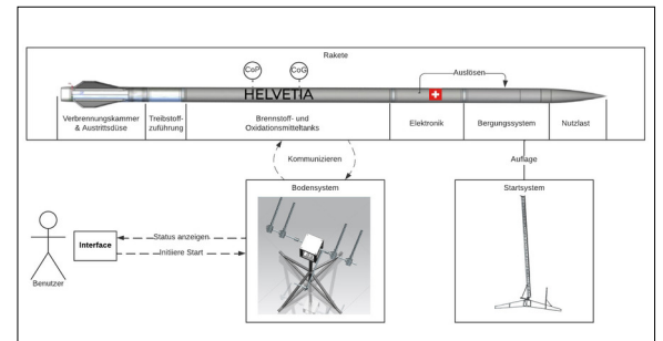
Abbildung 1: Kontextdiagramm Schwerpunkt Recovery Eigene Darstellung, ARIS Helvetia 2022 System
