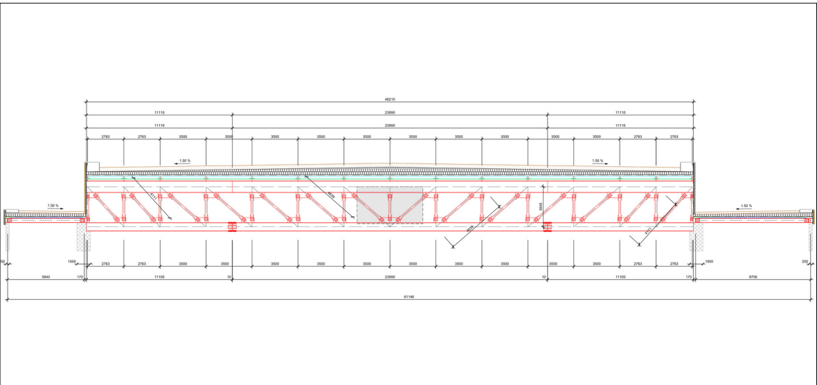
Querschnitt der Tragkonstruktion Eigene Darstellung
