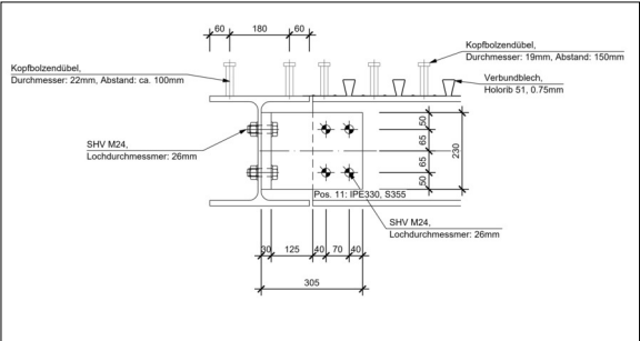
Detail Unterzugsverbindung Eigene Darstellung
