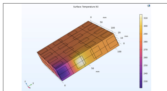
Temperaturverlauf bei Messungen mit Wärmeströmen auf zwei Messstempeln Eigene Darstellung
