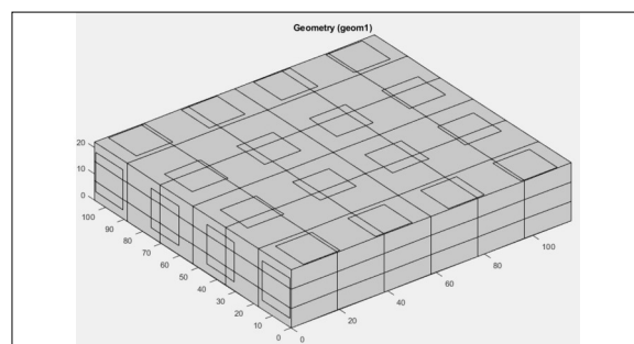
Geometrie mit Messstempel als Rechtecke auf der Oberfläche Eigene Darstellung
