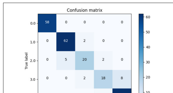
Abb. 2: Confusion Matrix für die Erkennung Eigene Darstellung
