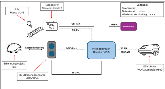
Schematischer Aufbau des Igelschutzmoduls Eigene Darstellung
