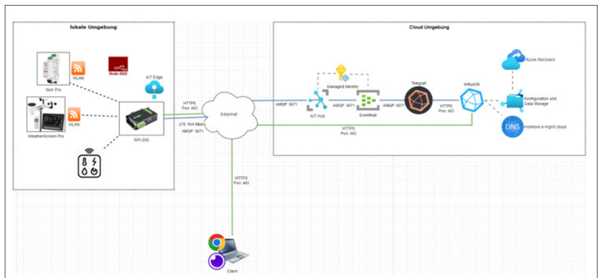
Systemarchitektur Eigene Darstellung
