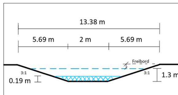
Aufweitung des Abflussprofils für grössere hydraulische Abflusskapazität Eigene Darstellung
