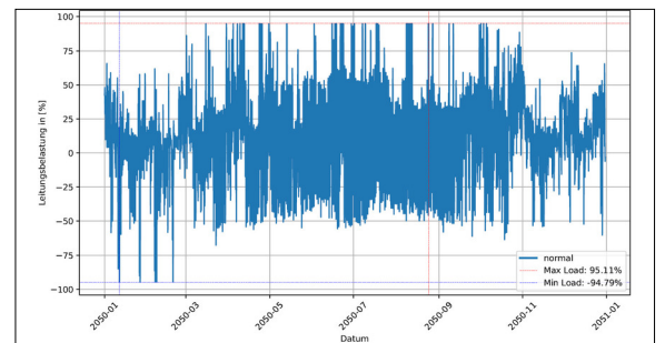
Leitungsbelastung einer 380kV Leitung Eigene Darstellung
