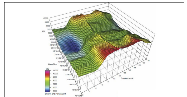
Stromnachfrage der Schweiz BFE/Swissgrid
