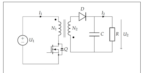
Übersicht über die gesamte Schaltung. Eigene Darstellung
