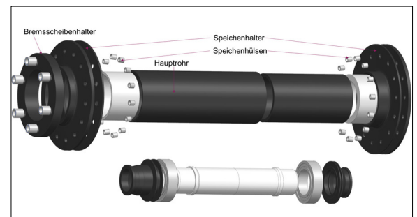
Einzelteile der Nabe Eigene Darstellung
