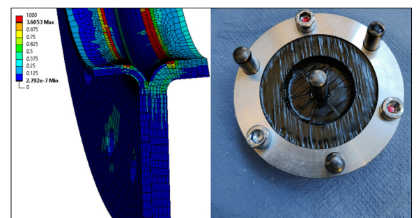
Kritische Stelle des Speichenhalters bezüglich Hashin und fertig drapierter Bremsscheibenhalter vor dem Aushärten Eigene Darstellung
