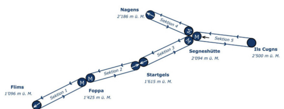
Gesamtnetz Ropetaxi-Projekt Flims Laax Falera (bereitgestellt durch Bartholet Maschinenbau AG, 2022)
