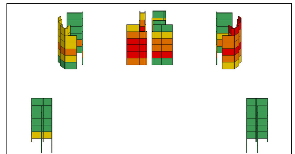
Ausnutzung Kerne Eigene Darstellung
