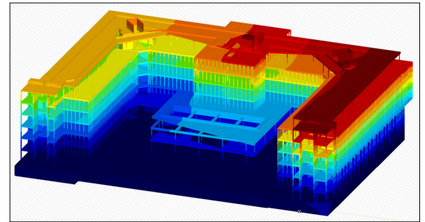
Erste Eigenschwingungsform (y-Richtung) Eigene Darstellung
