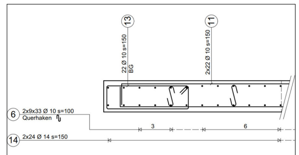
Bewehrung Randelement Erdbebenwand Eigene Darstellung
