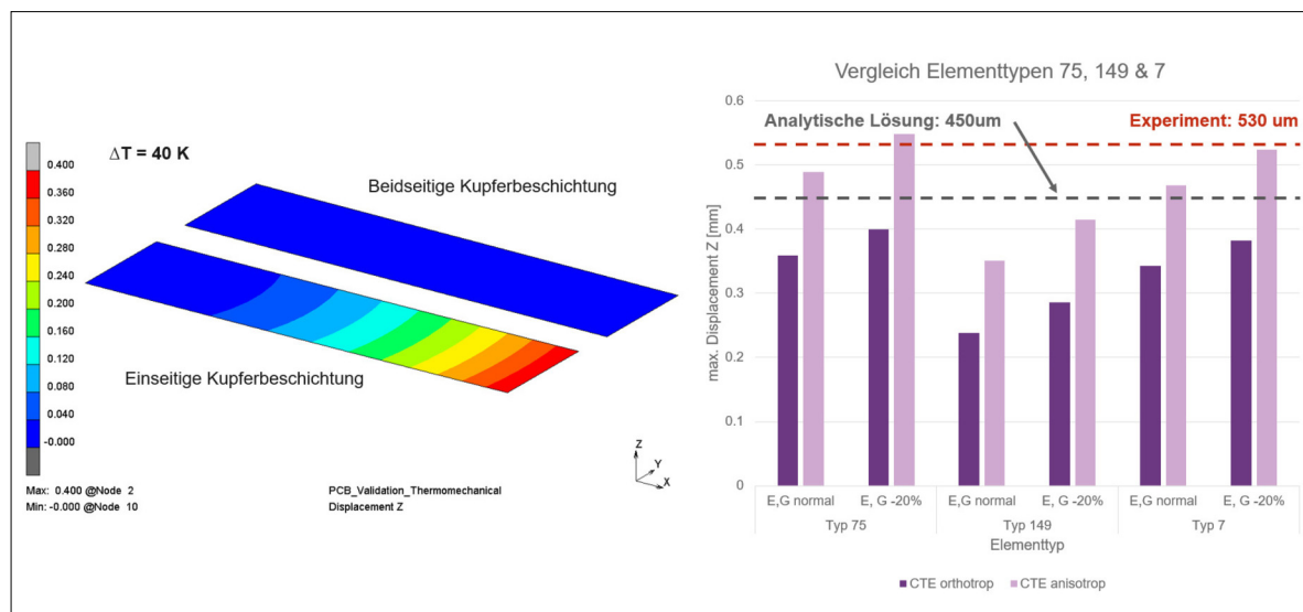
Simulation zur Validierung des thermomechanischen Verhaltens (Erwärmung PCB im eingespannten Zustand) Eigene Darstellung
