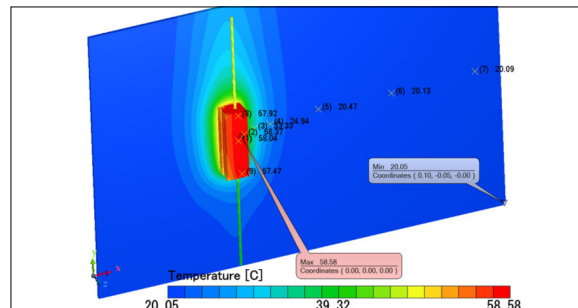
Simulation zur Validierung des thermomechanischen Verhaltens (Erwärmung PCB im eingespannten Zustand) Eigene Darstellung
