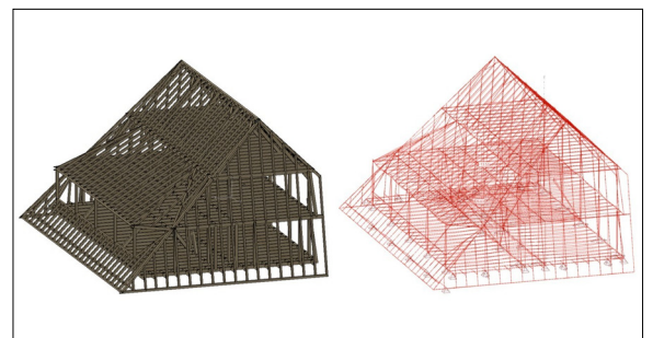
Stabtragwerk-Modell in ArchiCAD (li) und Cubus (re) Eigene Darstellung
