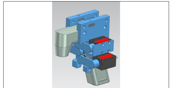
Prototyp im CAD Eigene Darstellung
