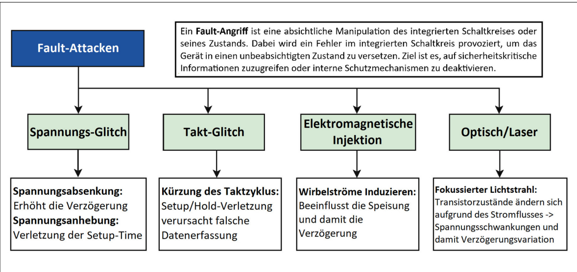
Übersicht über populäre Fault-Angriffe Basierend auf Buch "Hardware Security Training, Hands-on!"
