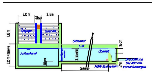
Abbildung 2: Fassung Schnitt Eigene Darstellung
