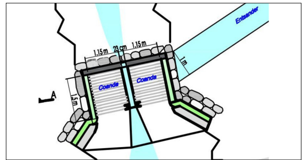
Abbildung 1: Fassung Grundriss Eigene Darstellung
