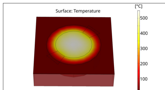
Simulation der Wärmeleitung und Temperatur des IR-Strahlers. IMP Institut für Mikrotechnik und Photonik
