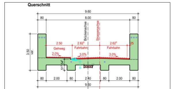
Querschnitt Spannbetonbrücke Eigene Darstellung
