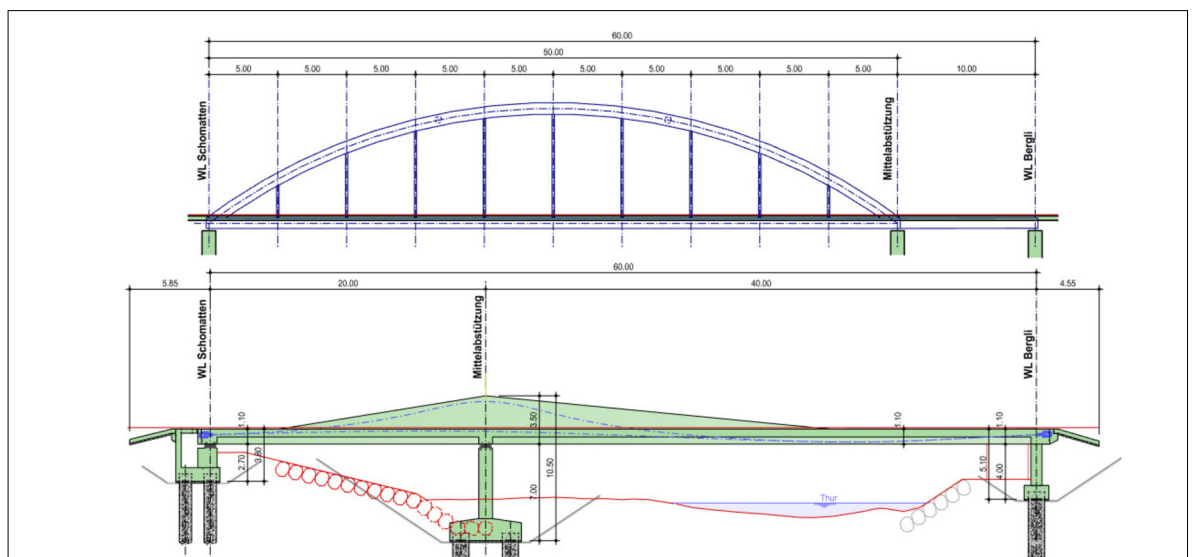
Variantenstudium: Stahlbogenbrücke und Spannbetonbrücke (Bestvariante) Eigene Darstellung
