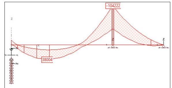
Momentenverlauf Spannbetonbrücke Eigene Darstellung
