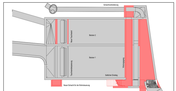
Grundriss des RüB Usterstrasse mit eingezeichneten Sanierungsvorschlägen Eigene Darstellung
