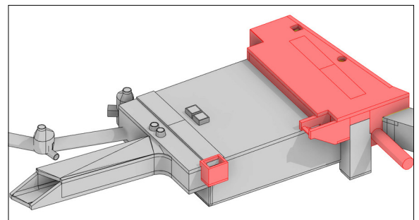
3D Ansicht mit der Deckenerhöhung und neuem seitlichen Einstieg Eigene Darstellung
