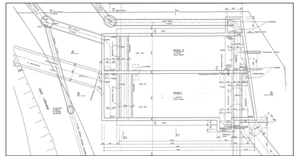
Ausschnitt aus dem PAW von 1988 PAW von Ingenieurbüro Gebr. Gossweiler
