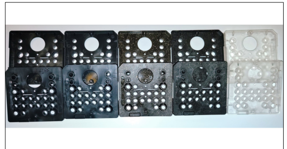
Vergleich technischer, nachhaltiger und preislicher Aspekte potenzieller Alternativwerkstoffen gegenüber HIPS Eigene Darstellung
