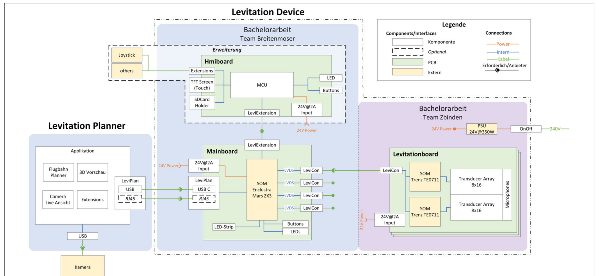
Abbildung 3: Übersicht Gesamtsystem: Blau hinterlegt sind alle Komponenten, die in dieser Arbeit umgesetzt wurden. Eigene Darstellung
