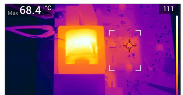
Temperaturoentwicklung nach 20 min Dauertest (400 V, 22.5 A, D = 0.5) Eigene Darstellung
