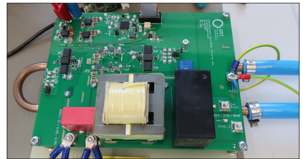
Bidirektionaler Buck/Boost-Konverter Eigene Darstellung
