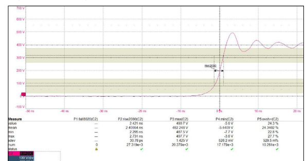
Messung am Switch-Node bei (400 V, 22.5 A, D = 0.5) Eigene Darstellung
