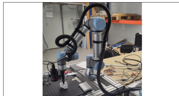
Montiertes Kamerasystem Eigene Darstellung
