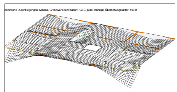
Verformung der Balkenecke im quasi-ständigen Lastfall Eigene Darstellung
