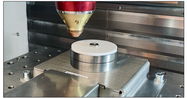
Integrierte Drehachse in der LMD-Maschine Eigene Darstellung
