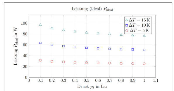
Abbildung 1: Ideale Verdichterleistung als Funktion des Druckes p_1 (siehe Abb. 2) für verschiedene Temperaturerhöhungen Eigene Darstellung
