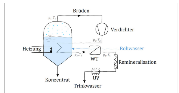
Abbildung 2: Schematische Darstellung einer möglichen Brüdenverdichtung zur Trinkwasseraufbereitung Eigene Darstellung
