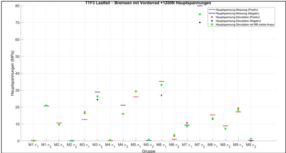
Beispiel für den Vergleich der Hauptdehnungen Eigene Darstellung
