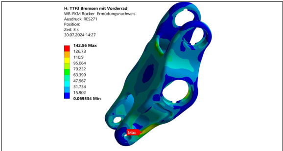
Rocker – Kritischer Bereich an der Dämpferanbindung Eigene Darstellung
