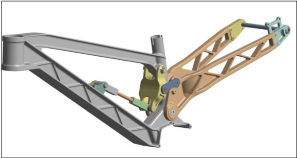
FEM-Modell des Mountainbike-Rahmens für die Analyse Eigene Darstellung
