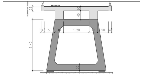
Querschnitt des Brückenober- und Unterbaus Eigene Darstellung
