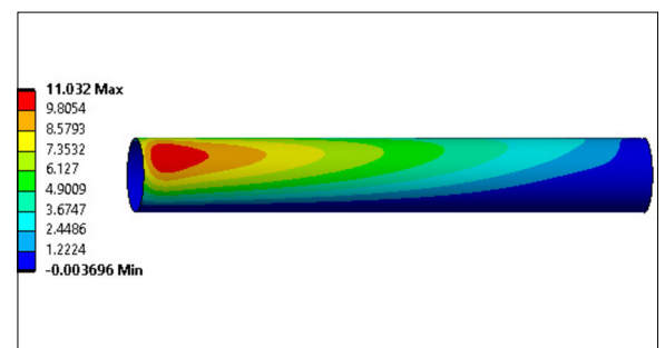
Erste Hauptspannung in MPa an einem Biegebelasteten Rohr mit abwechselnden 10° und -10° Faserwinkelausrichtungen Eigene Darstellung
