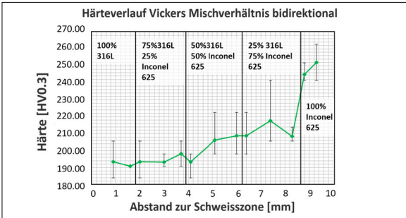
Vickers Härteverlauf Mischverhältnisversuch von Stahl 316L und Inconel 625 Eigene Darstellung
