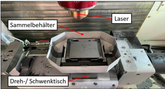
Hybridmaschine mit montiertem Sammelbehälter Eigene Darstellung
