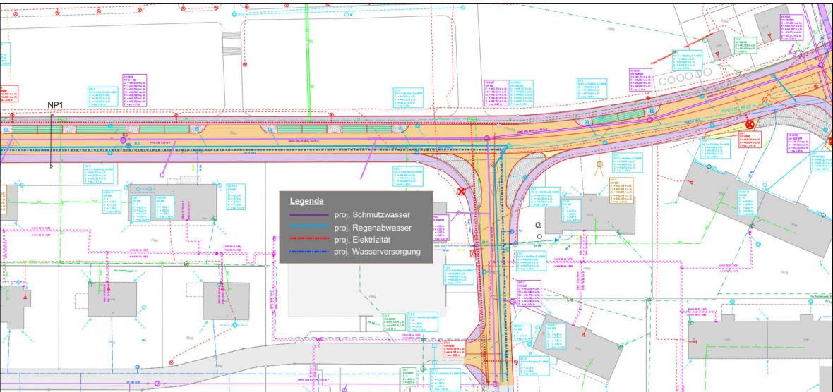
Situation Werkleitungen Eigene Darstellung
