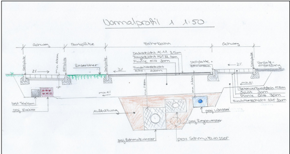
Normalprofil 1:50 Eigene Darstellung
