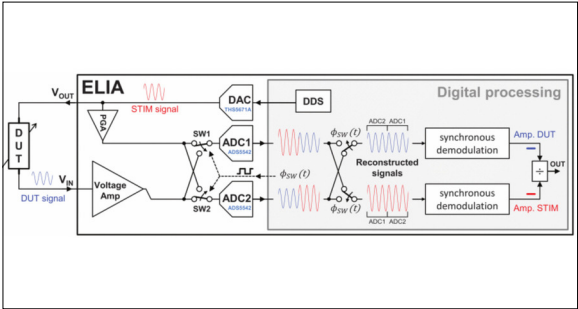
ELIA Structure doi: 10.1109/ICECS.2016.7841146
