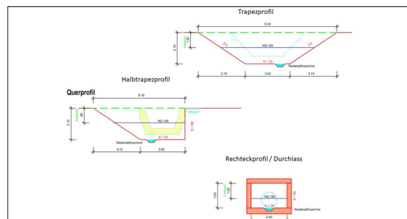
Abbildung 2 - Drei Querprofile des Variantenstudiums Eigene Darstellung
